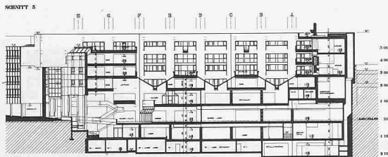
Längsschnitt durch Innenhof
