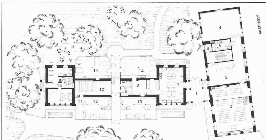
Erdgeschoss, Institut.
