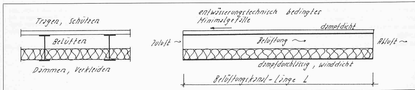
Bild 1. Schnitte durch ein durchlüftetes Kalddach. Links: Querschnitt, rechts: Längsschnitt
