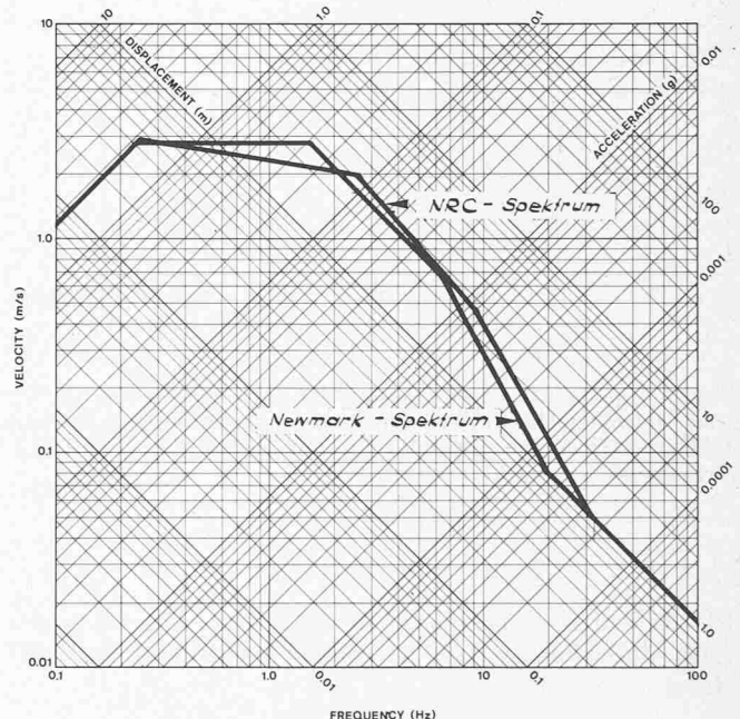
Bild 16. Bemessungsspektren. Horizontale Bemessungsspektren (Mittelwert plus eine Standardabweichung) für Lockergestein und verwitterten Fels, skaliert auf 1.0 g Horizontalbeschleunigung, Dämpfung \beta = 5 Prozent
