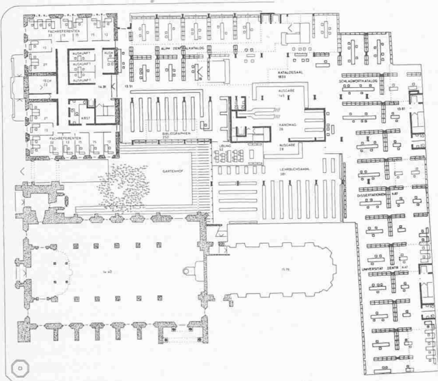
Grundriss Ebene Katalogsaal 1:1100
