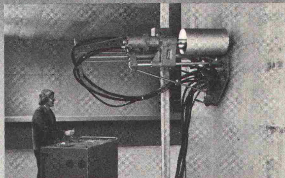
Bohren und Fräsen mit dem gleichen Pumpenaggregat
