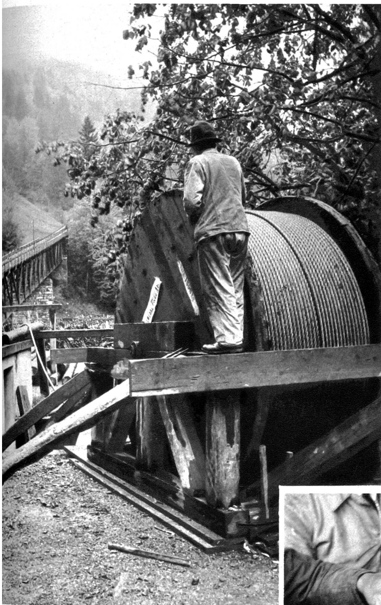
Von der Rolle wird das neue Seil hinaufgezogen; doch vorher wird der Seilkopf hergestellt
