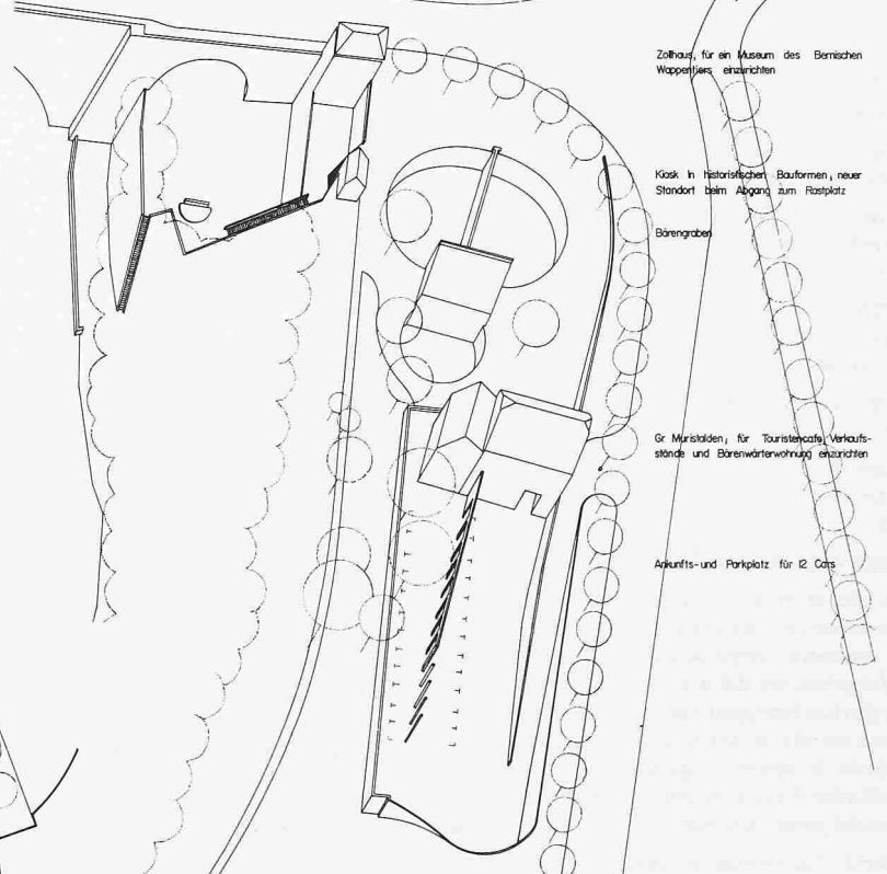
Grundriss Ebene 520.00, 1:1500
