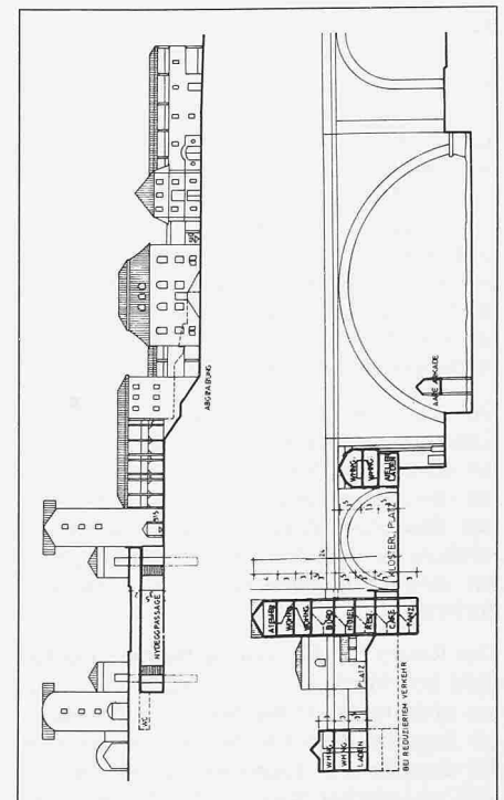
Schnitt Nydegpassage/Ansicht 1:1500
