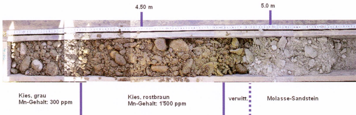
Fig. 17: Bohrkern Kb 12/1 (Tiefenbereich 4–5.5 m u. T.); rostbraune Verfärbung infolge Bildung von Mn-Oxid [semiquantitative Analysedaten aus mobiler XRF].
