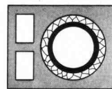
Doppelzuger mit Ventilationsschacht Elementhöhe 33 cm
