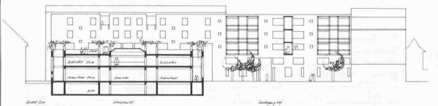
Schnitt/Ansicht Rosshofgasse-Platz 1:850
