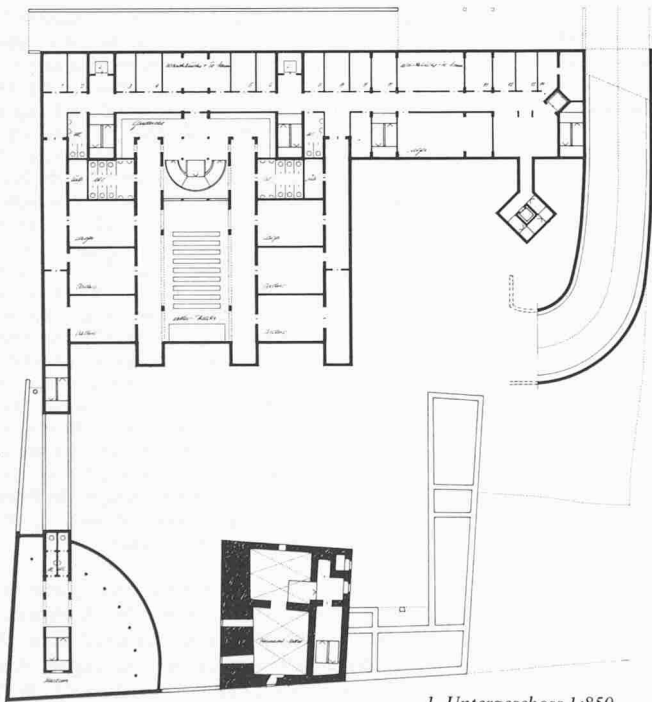
1. Untergeschoss 1:850
