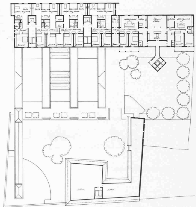
3. Obergeschoss 1:850
