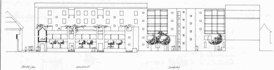
Ansicht von Osten, Seminartrakt 1:850
