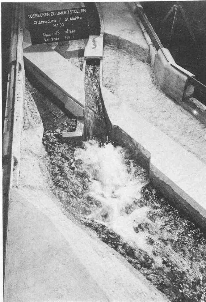
Bild 8. Aufnahme des Tosbeckens der Umleitung des Inns im Modell (Massstab 1:30). Die Energieumwandlung des aus dem Stollen schiessenden Strahls wird durch die im Tosbecken eingebauten Rehbockzähne wesentlich verstärkt
