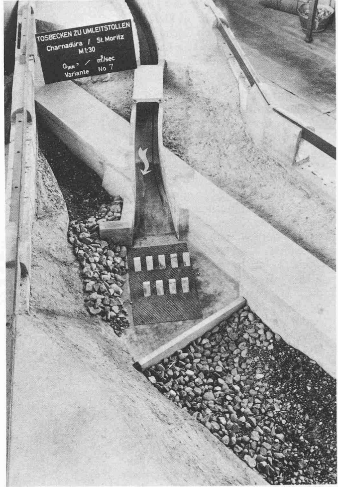
Bild 8. Aufnahme des Tosbeckens der Umleitung des Inns im Modell (Massstab 1:30). Die Energieumwandlung des aus dem Stollen schiessenden Strahls wird durch die im Tosbecken eingebauten Rehbockzähne wesentlich verstärkt
