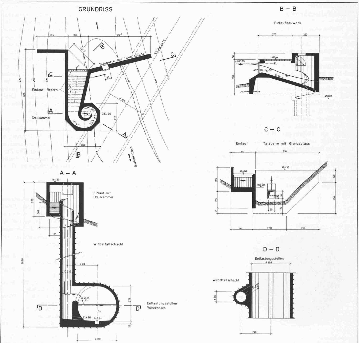
Bild 14. Verzeichnis der Bauwerke der Büttenebäche, bestehend aus Rückhaltebecken, Talsperrenabschluss und Einlaufbauwerk des Wirbelfallschachtes
