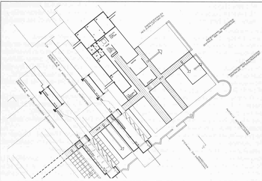
Lageplan 1:2500
