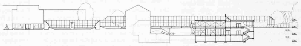
Schnitt 3-3 1:500
