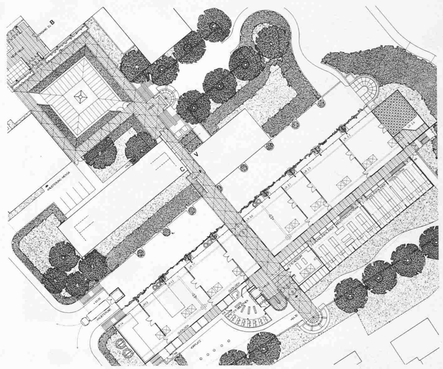
Grundriss Erdgeschoss 1:500
