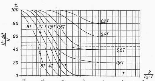
Bild 6. Darstellung des zeitlichen Verlaufes der Sickerlinie im Stützkörper während und nach einer vollständigen Absenkung des Stauspiegels (ausgehend von Vollstau). Böschungseignung des Stützkörpers 1:2,08. Böschungseignung des Kernes 1:0,16. Durchlässigkeitsverhältnisse: Kern und Untergrund im Verhältnis zum Stützkörper sehr klein
