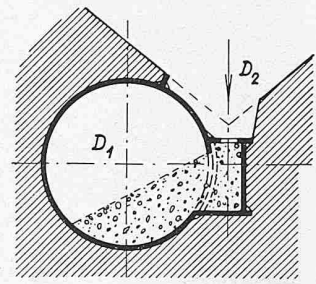
Bild 3. Querschnitt C-C des Sandabzugsrohres, stark vergrössert
