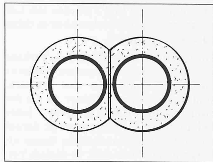
Bild 2. Zusammengerückte Leitungen
