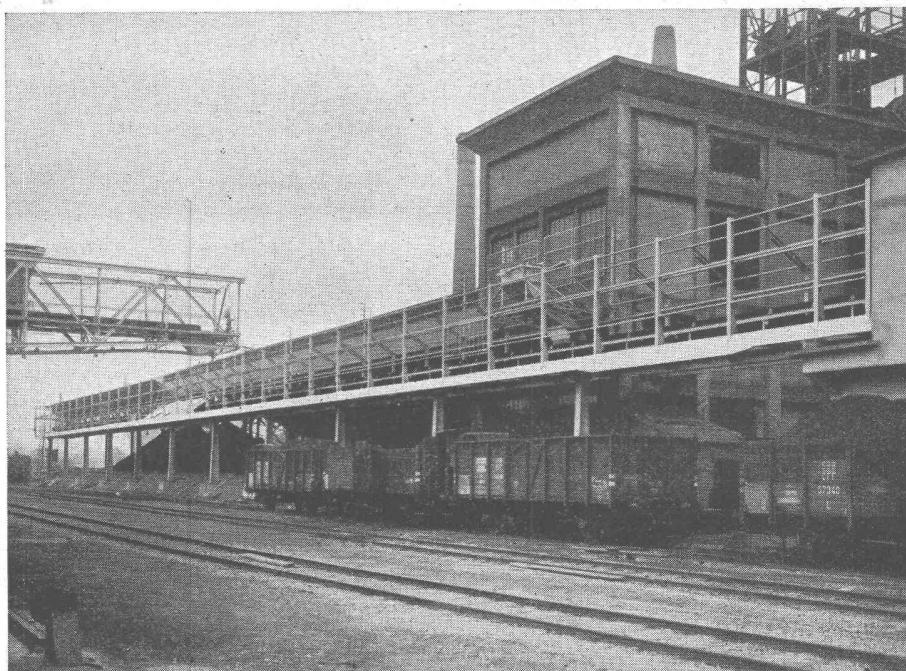
Förderband-Passerelle Länge 115 m
