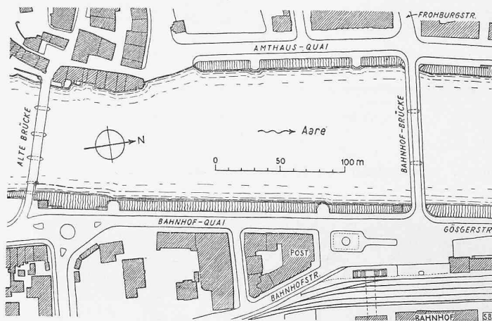
Bild 1. Lageplan, Masstab 1:4000
