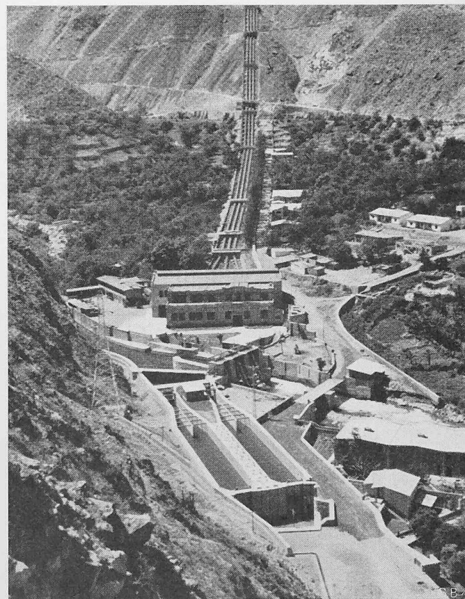
Bild 12. Entsander (im Vordergrund) und Wasserfassung für das Kraftwerk Moyopampa, darüber Zentrale und Druckleitung der obren Stufe.
