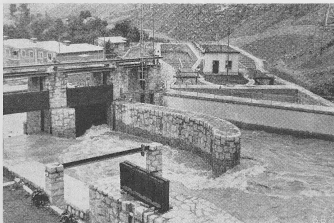
Bild 11. Wasserfassung für das Kraftwerk Moyopampa. Man beachte das abgeboogene obere Ende der Trennmauer.
