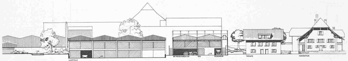
Ansicht von Osten 1:900, Schweineställe, Lager/Maschinentrakt, Werkstatt-Trakt, Therapie, Heimzentrum
