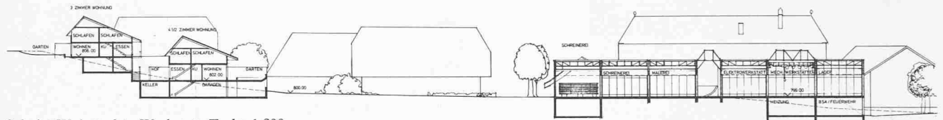
Schnitt Wohntrakte-Werkstatt-Trakt 1:900
