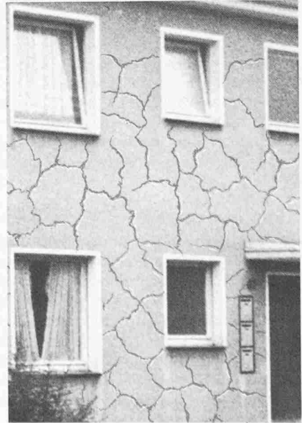
Bild 3. Spannungsrisse
