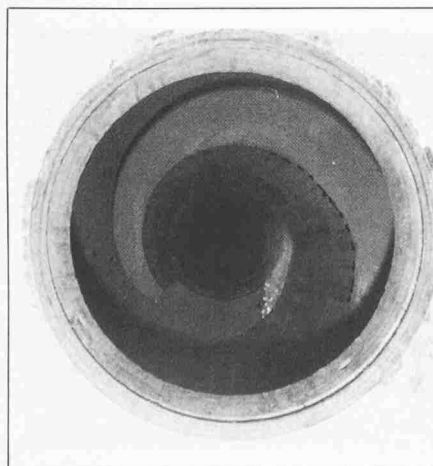
Bild 10. Spiralförmiger Einlauf des Wirbelfallschachtes
