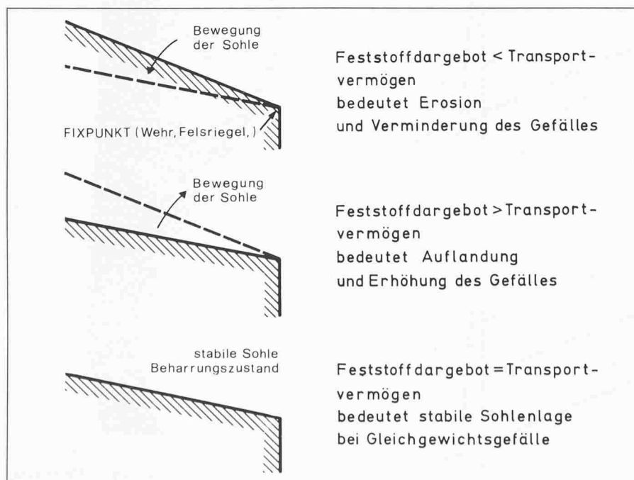
Bild 1. Drei schematische Längsschnitte eines Flusslaufes. Entwicklung des Sohlengefälles bei Erosion (oben) und bei Auflandung (Mitte). Beharrungszustand zwischen Feststoffdargebot und Transportvermögen (unten)
