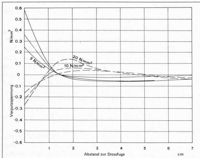
Diagramm 7 (Fugenbereich). Verputzspannungen in Abhängigkeit zum Abstand zu einer Stossfuge in der Wärmedämmung bei unterschiedlichen Elastizitätsmoduln (5, 10 und 20 N/mm 2 ) der Wärmedämmung unter 0,1% Schwinden der Wärmedämmung.
