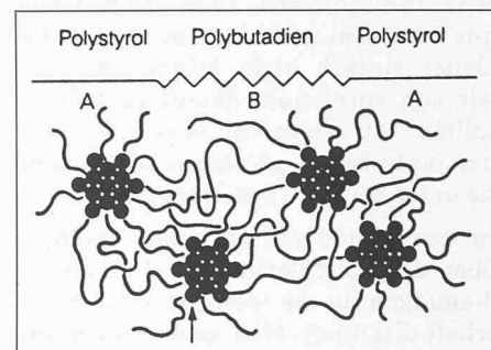
Bild 3. SBS (ABA) und Elastomerbitumenstruktur
