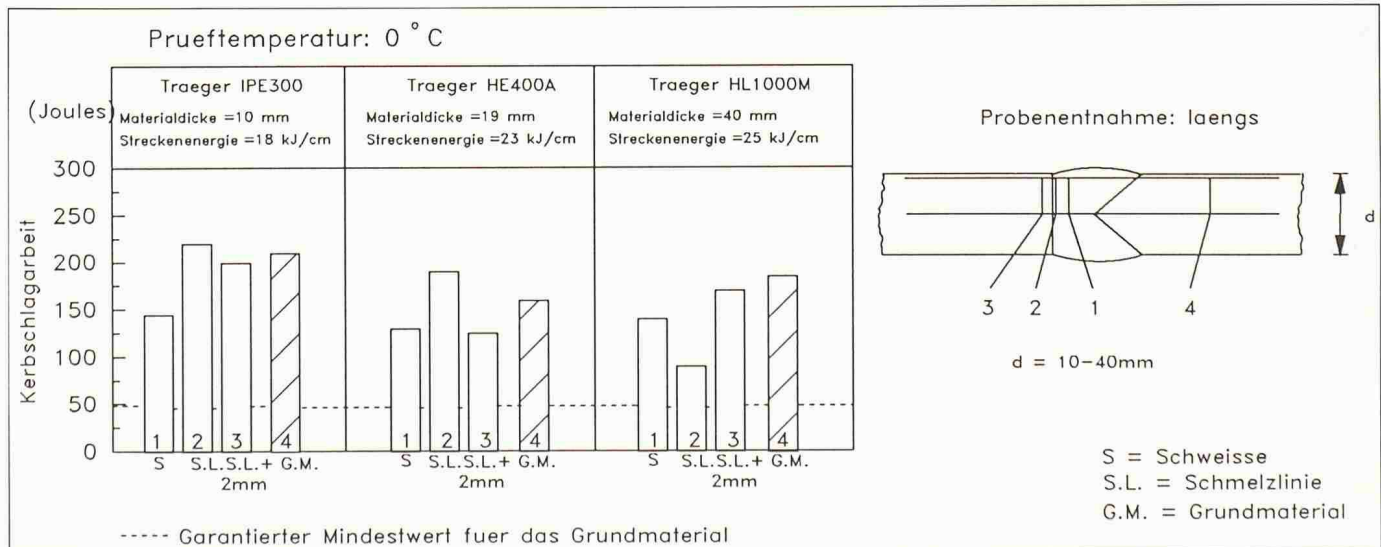
Bild 5. Charpy V-Kerbschlagbiegeversuch auf einer Lichtbogen-handgeschweissten Schweisverbindung
