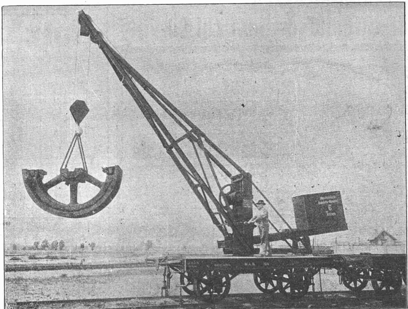
Fahrbarer Wagendrehkran mit Handbetrieb zum Einstellen der Eisenbahnzüge; geliefert u. A. für Essen, Luxemburg, Leipzig, Zürich.
