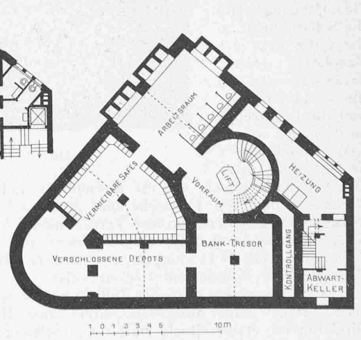
Abb. 1 und 2. Grundrisse vom Kellergeschoss, Halbstock und Erdgeschoss der Eidg. Bank in St. Gallen. — Masstab 1 : 400.
