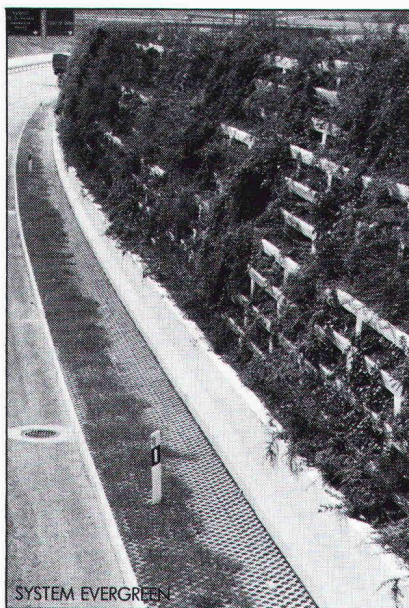
Bepflanzte Raumgitterwand
