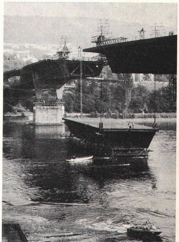
Hochheben des 650 Mp schweren Mittelteils der Horschheimer Rheinbrücke bei Koblenz.
