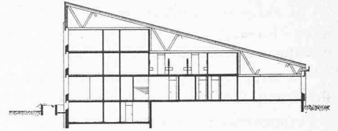
Schnitt Offiziersunterkunft 1:650
