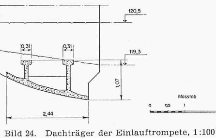
Bild 24. Dachträger der Einlauftrumpete, 1:100
