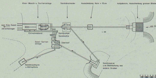
Grundriss der Kies-Sand-Aufbereitungsanlage
