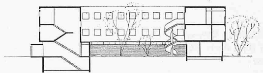
Schnitt 1:700 durch Gefängnishof
