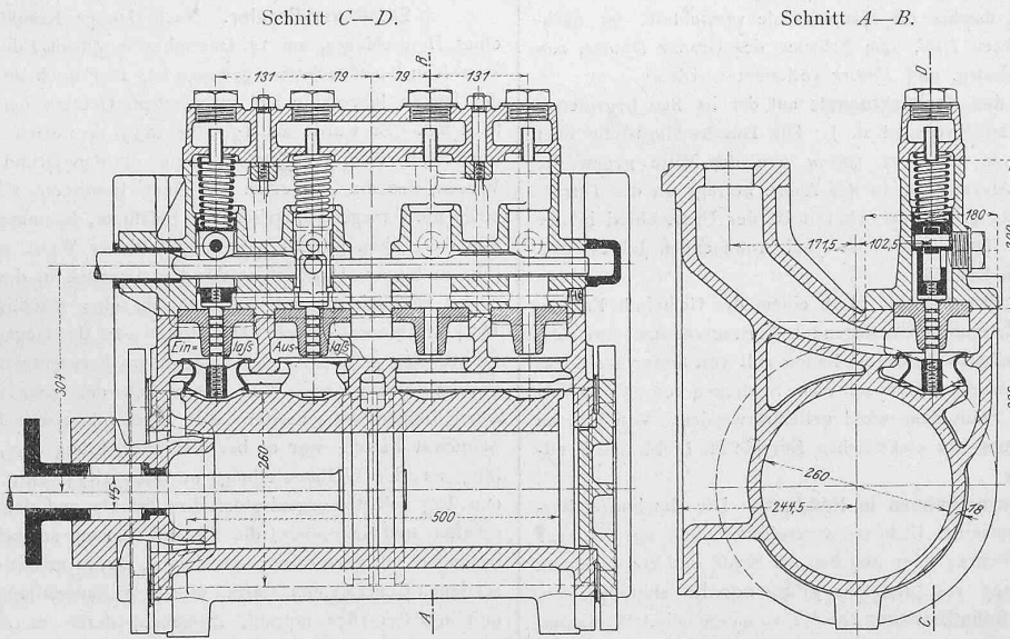
Lokomotivzylinder mit Ventilsteuerung. — Masstab 1 : 10.
