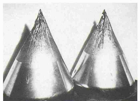
Sanderosionsschäden an Pelton-Düsen-nadeln: Aufprallbeschleunigungen der Sandkörner bis 6500 g
