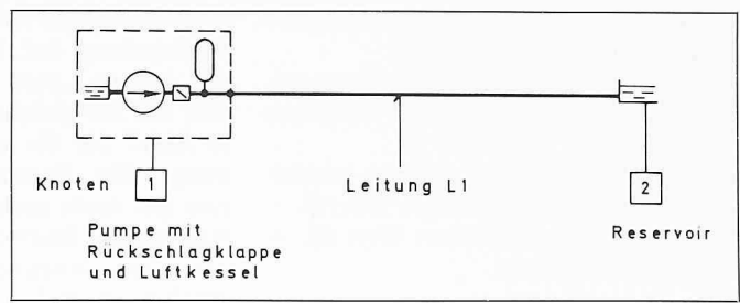
Bild 12. Anlage Lyren. Mathematisches Modell
