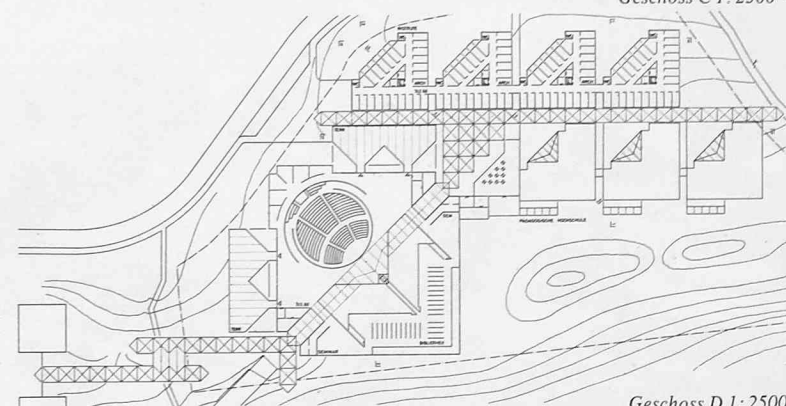
Geschoss D 1: 2500
