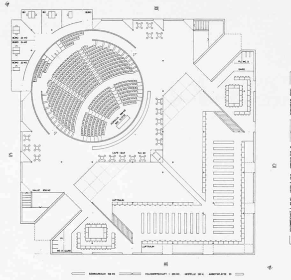
Geschoss D, 743.60, 1:900
