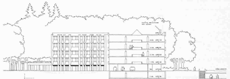
Schnitt Halle 1:1000
