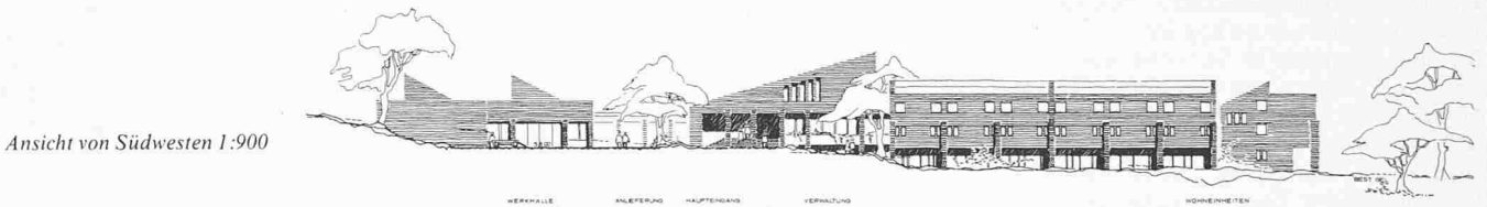
Schnitt Werkhalle 1:900
