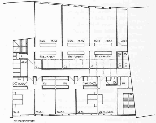
Grundriss 3. Obergeschoss 1:400
