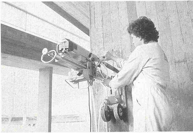
Bild 3. Probeentnahme für Chloridbestimmung mittels Diamantbohrung (Werkphoto SIKA AG)
