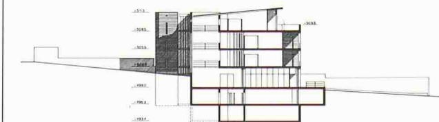
sezione trasversale
