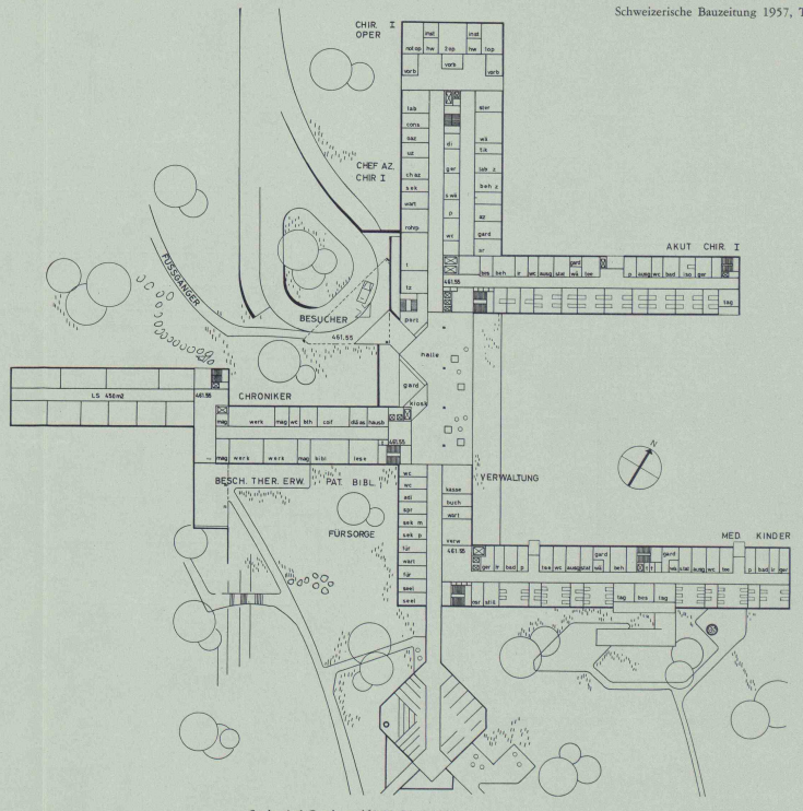
Stadtspital Geschoss 461.55, M. 1:1000
