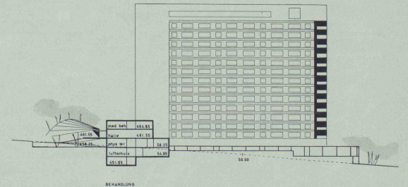
Stadtspital Südost-Ansicht Bettenhaus, M. 1:1000
