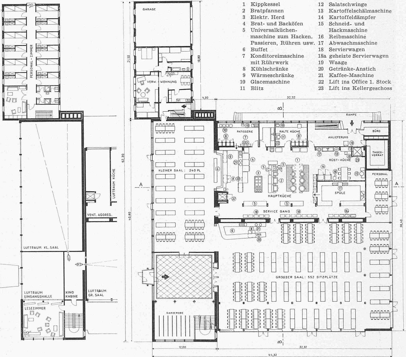
Zwischengeschoss
