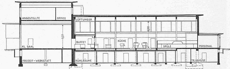
SCHNITT A-A
