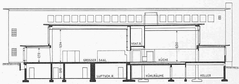
SCHNITT B-B
