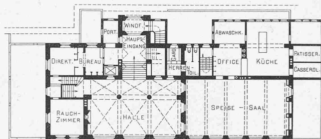
Abb. 2, 3, 4, 5. Grundrisse vom Erdgeschoss, Zwischengeschoss, Hauptgeschoss und I. Obergeschoss.
