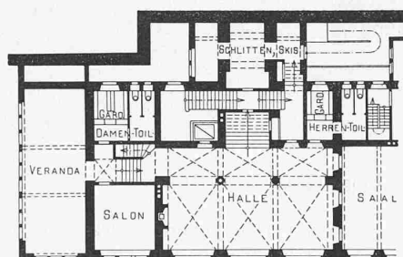
Abb. 2, 3, 4, 5. Grundrisse vom Erdgeschoss, Zwischengeschoss, Hauptgeschoss und I. Obergeschoss.
