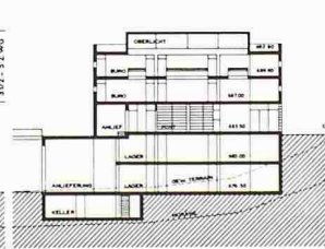
Längsschnitt Post C-C
