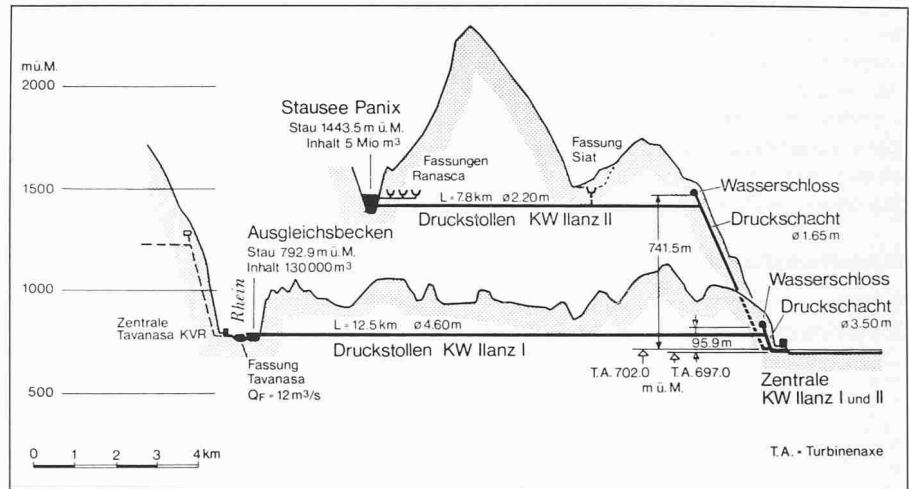
Bild 2. Längenprofil
