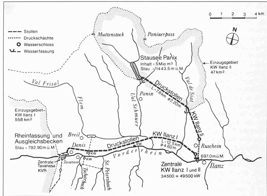
Bild 1. Übersichtskarte Kraftwerke Ilanz I und II
