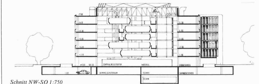
Schnitt NW-SO 1:750
