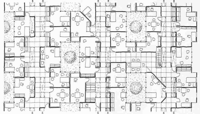
Größere Einzelebene - 10,5 - 15 qm /Arbeitspl.
