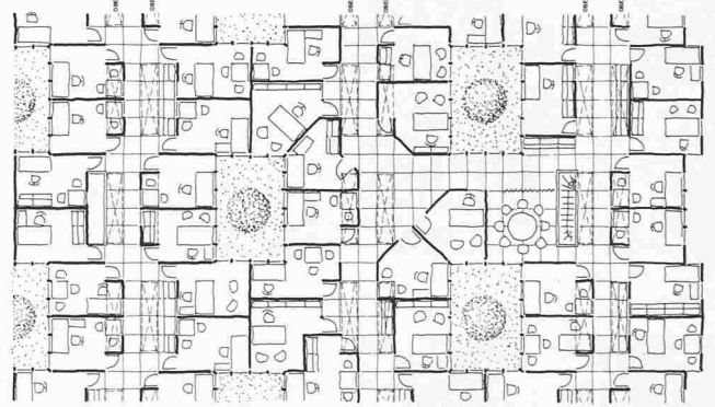
Oben links: Unterteilung und Möblierung, Kombinationsmöglichkeiten, Ausschnitt EG
