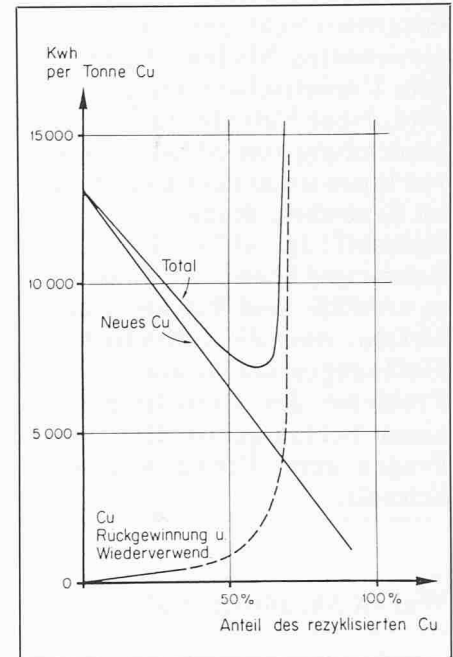
Bild 2. Energieaufwand für die Herstellung einer Tonne Kupfer in Abhängigkeit des prozentualen Anteils an rezykliertem Kupfer (Stumm und Davis 1974, [6])
